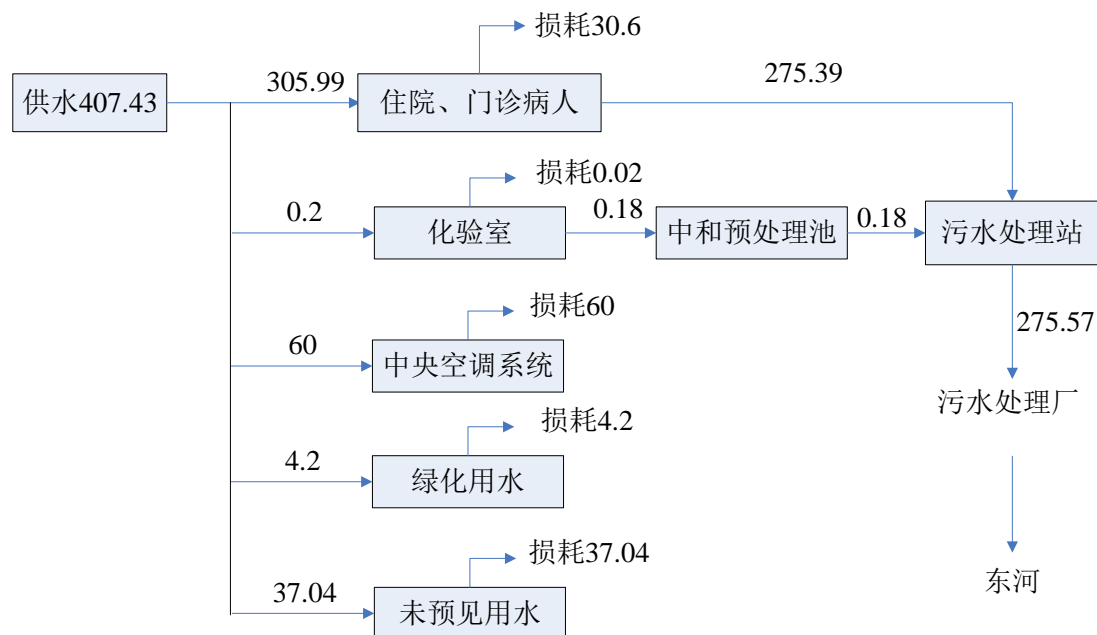
图4.2-3 全院水平衡图 (单位: t/d)
