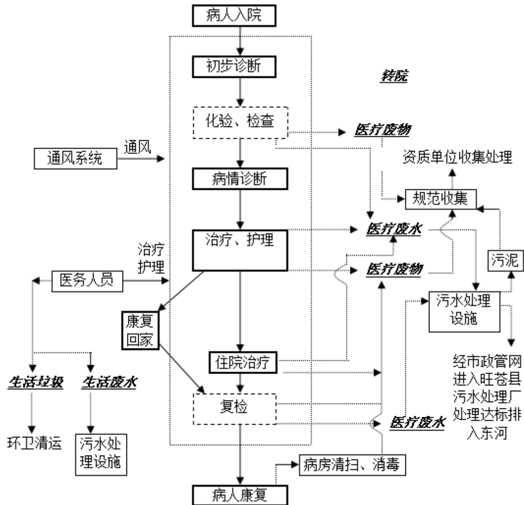
4.2-1 营运期工艺流程及产污环节图
